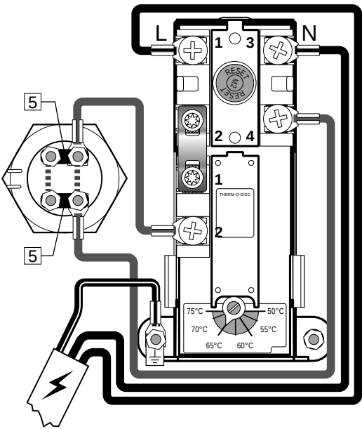
Kytentäkaavio
