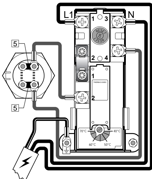
Elslutning, schematisk
